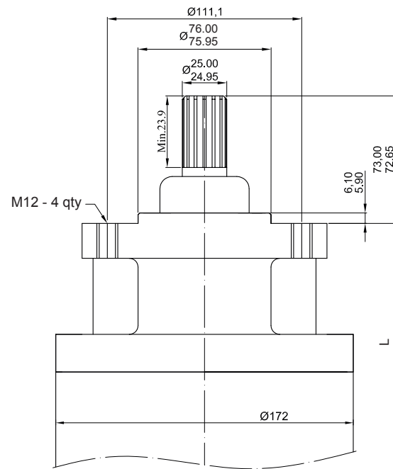
Motor 7"
