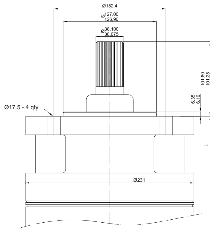
Motor 10"
