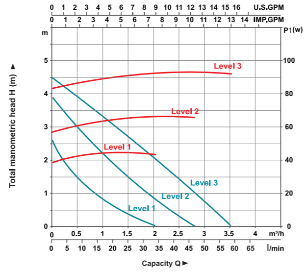
LRP32-50/180 — Q-H — Q-P
