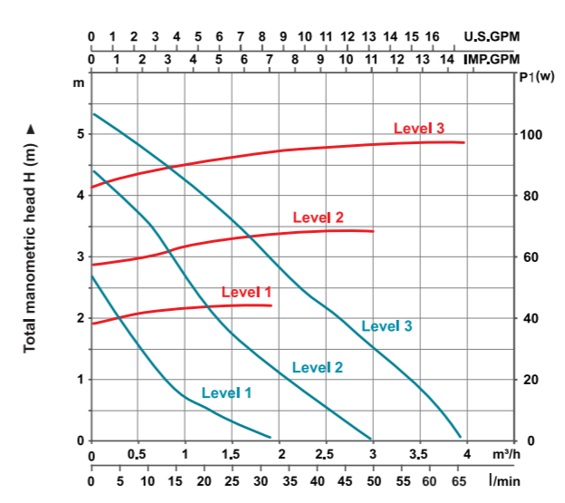
LRP25-60/180 — Q-H — Q-P
