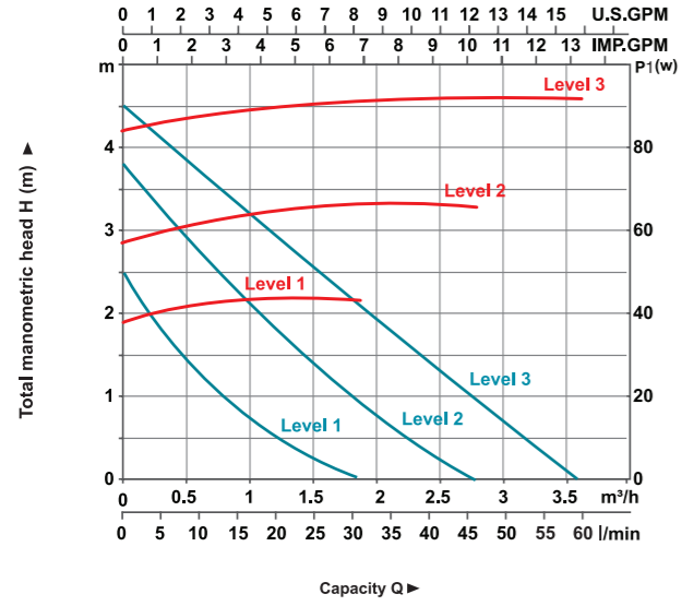
LRP25-50/180 — Q-H — Q-P
